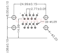
PCB布局 (PCB Layout)
