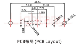
PCB布局 (PCB Layout)
